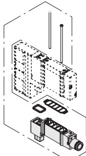
Höhenverkettung
