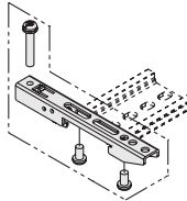
DIN-Schienenbefestigung
